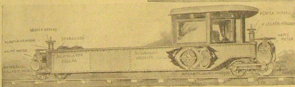
Brennan egysínű vasútjának kocsija.
