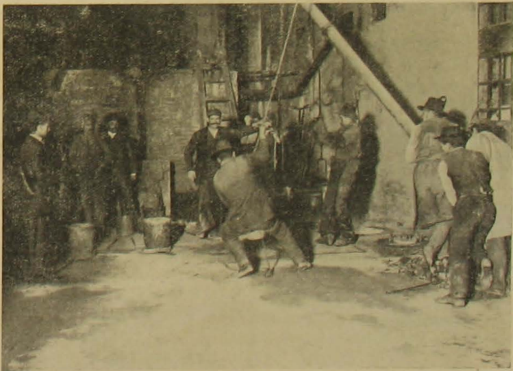
Az 1200 fokra hevített bronzot daruval kiemelik az olvasztó kemenczéből.
