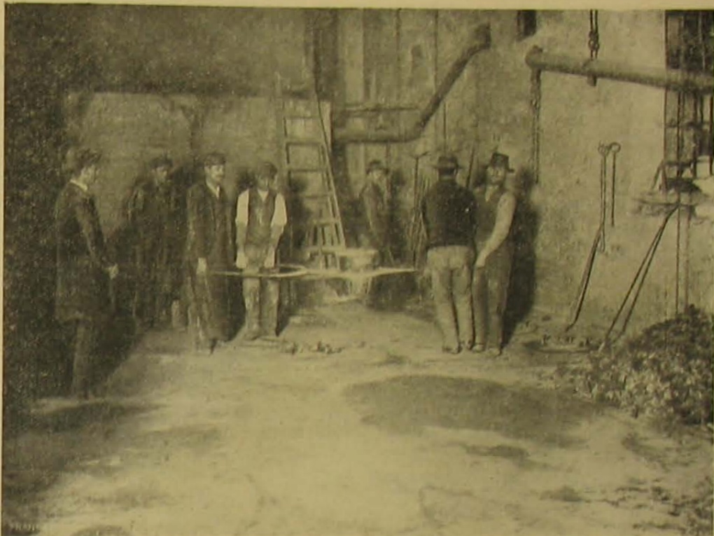
Az olvasztott bronzet graphit-tégelyben a súlyasztó gödörben levő formába hoz visszük.
