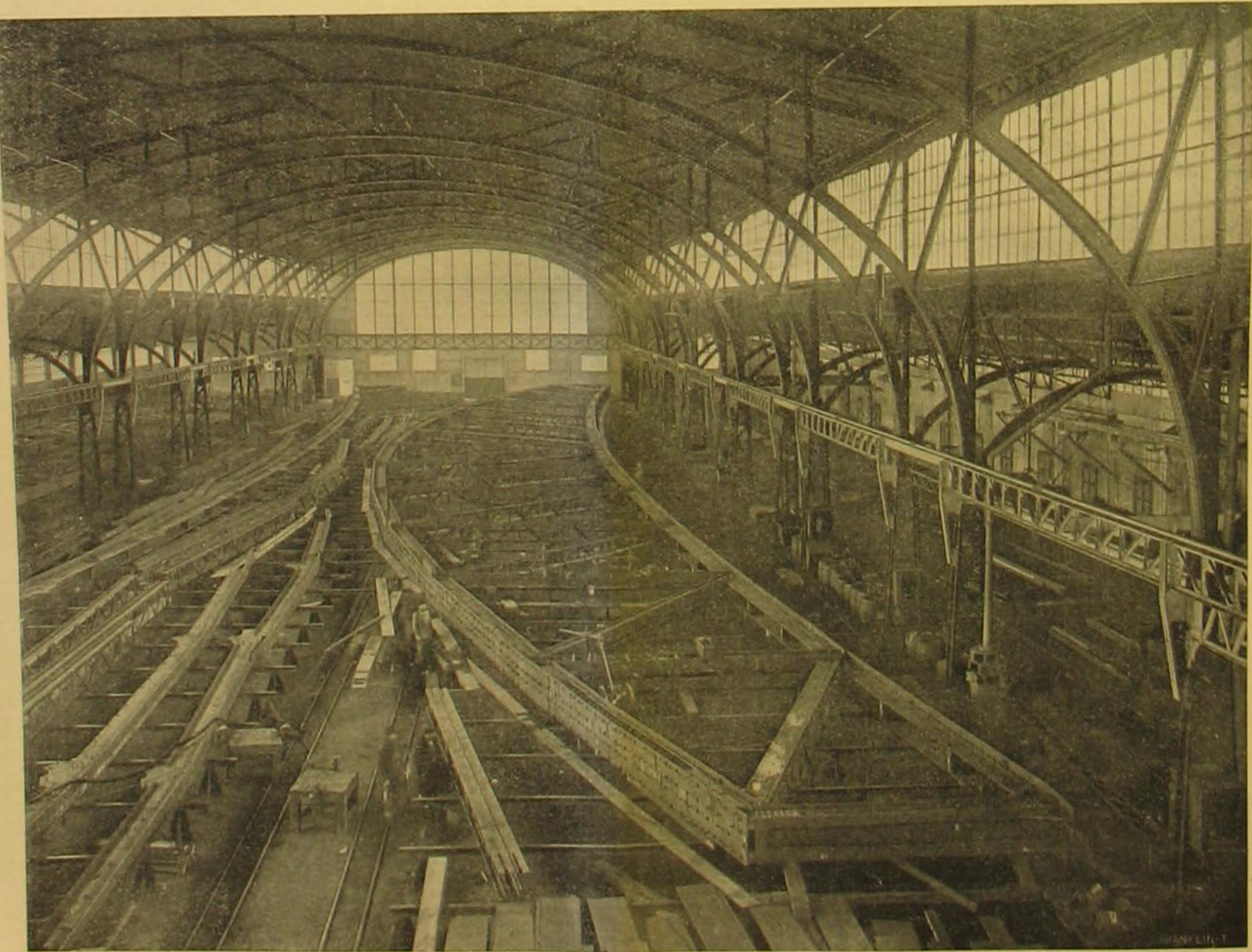
A baja-bátsági Dunahíd építése. A híd-szorkozot építő az államvasutak budapesti gőpgyárában.
