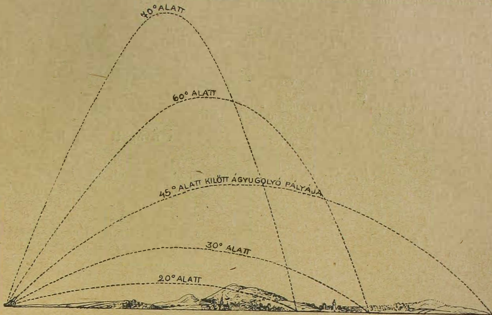
A lövedék pályája különböző emelkedések alatt.
