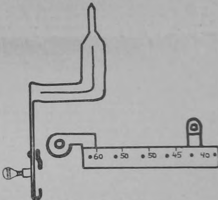
35. ábra: A célzótűske és az irányzósín.
