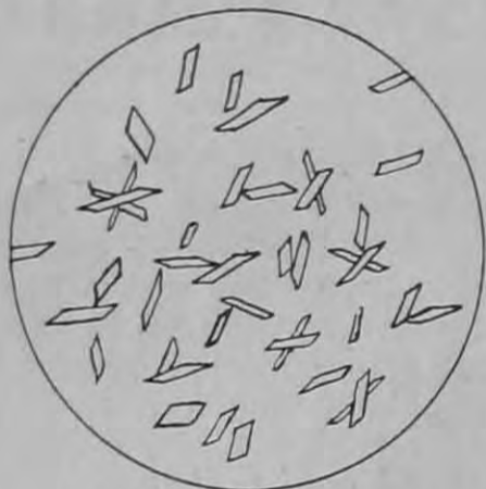
5. ábra: Haemin jegecek.
