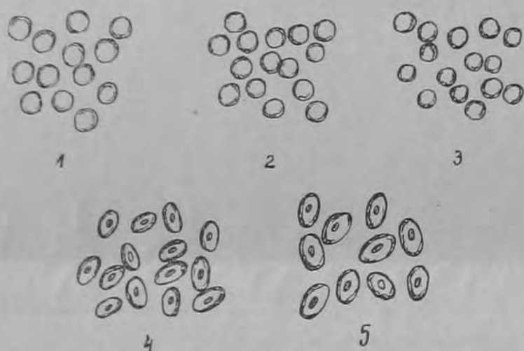
6. ábra: Vörös vértestek. 1 Ember. 2. Disznó. 3. Tengeri malac. 4. Tyuk. 5. Csuka.
