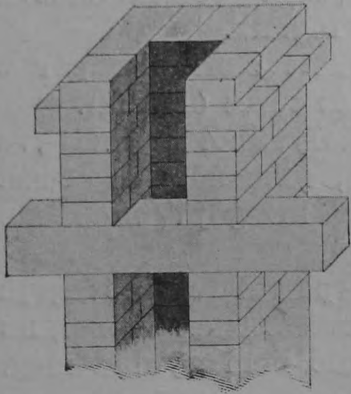
10. ábra. Beépített gerenda.
