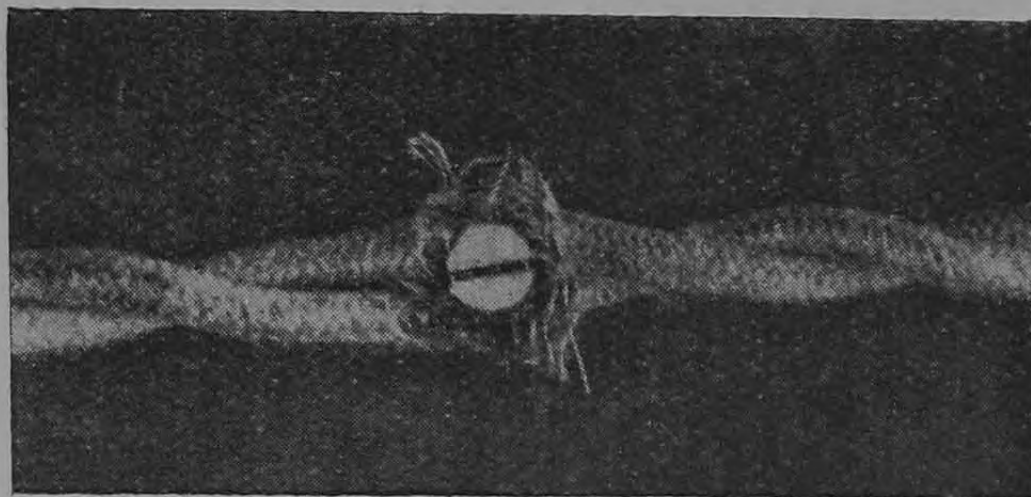
11. ábra. Rövidzárlat oka szemléltetően ábrázolva: vezeték közé vert szög.
