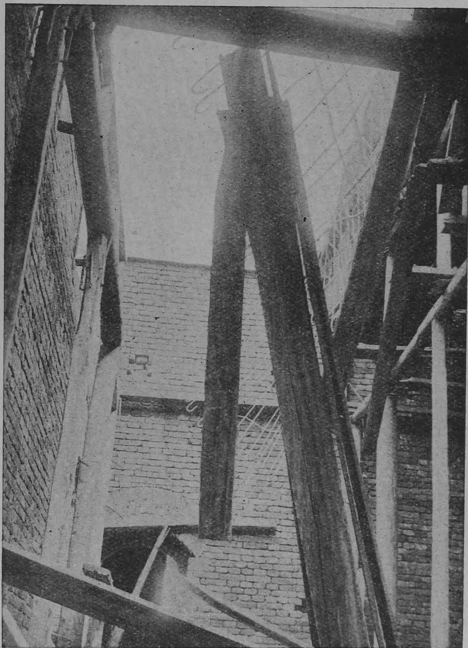
29. ábra. Helyszini felvétel építkezési balesetknél. Összeomlott betonépítkezés.
