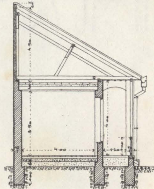
A-B Metszet. 1:100.
