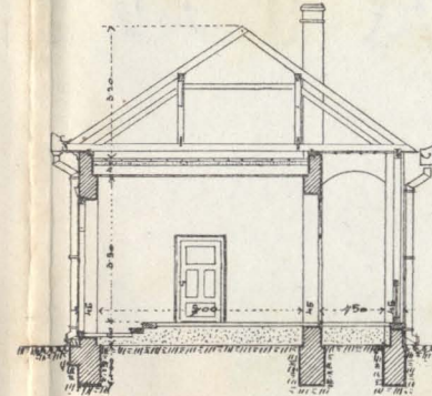
C-D Metszet. 1:100.
